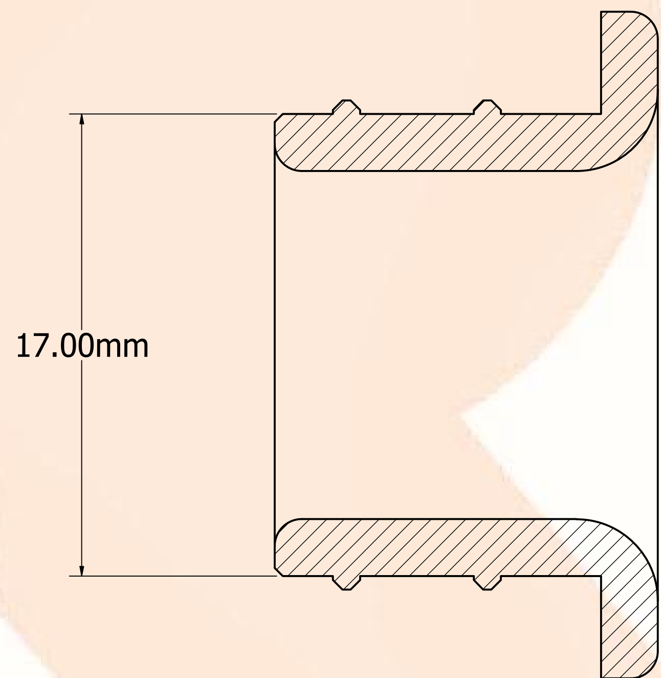
SECTION A-A SCALE 7 : 1
