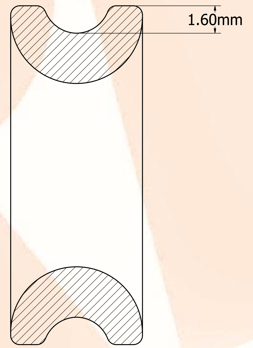
SECTION A-A SCALE 10 : 1
