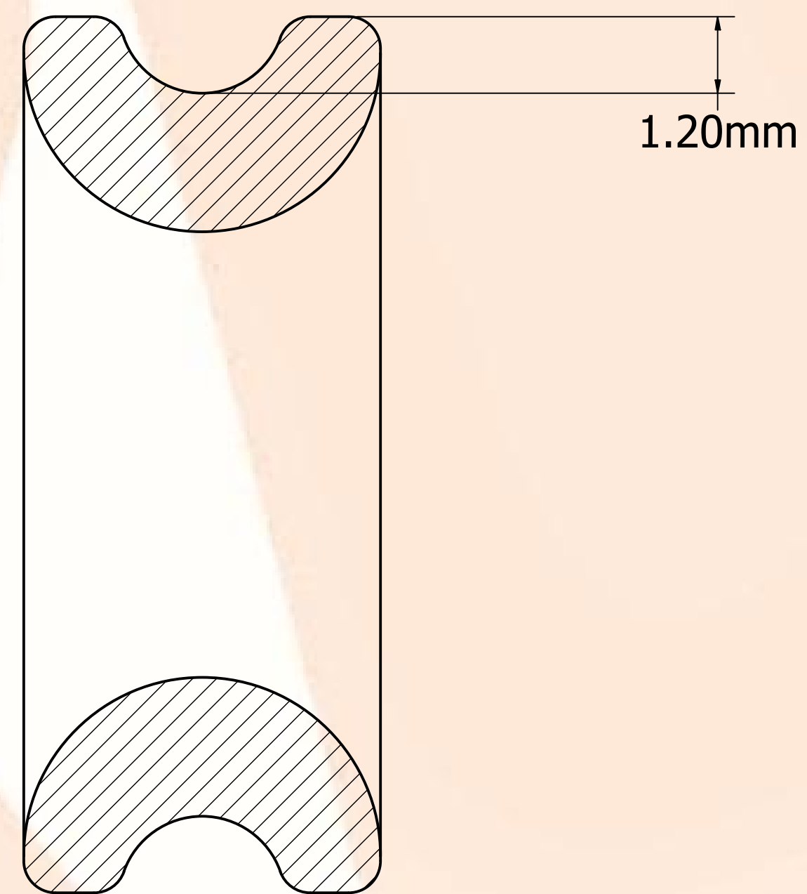
SECTION A-A SCALE 12 : 1
